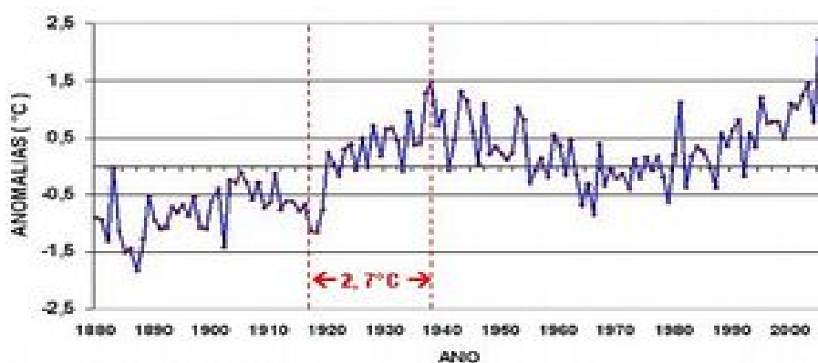
Figura 2. Anomalias de temperatura do ar no Ártico entre 1880 e 2004 (Fonte de dados: http://www.giss.nasa/data/gistemp , 2007).
