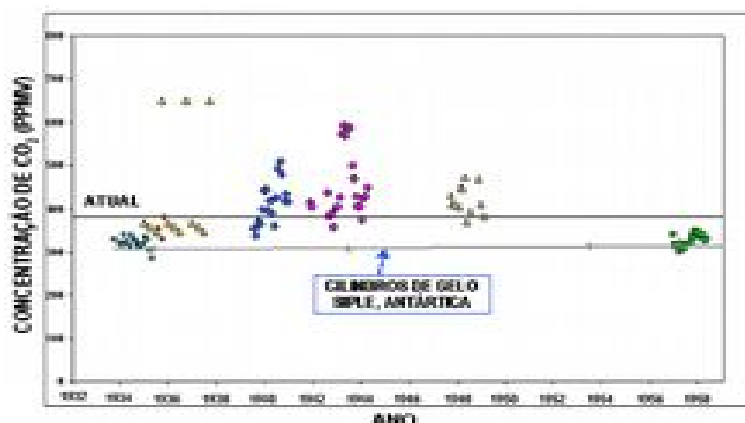
Figura 4. Medições químicas de CO 2 atmosférico, feitas por vários pesquisadores na primeira metade do Século XX, antes do início das medições em Mauna Loa, Havaí, em 1957/58.
